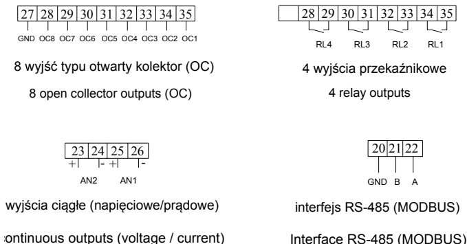
Rys. 4: Sposób połączenia sygnałów wyjściowych w zależności od kodu wykonania
